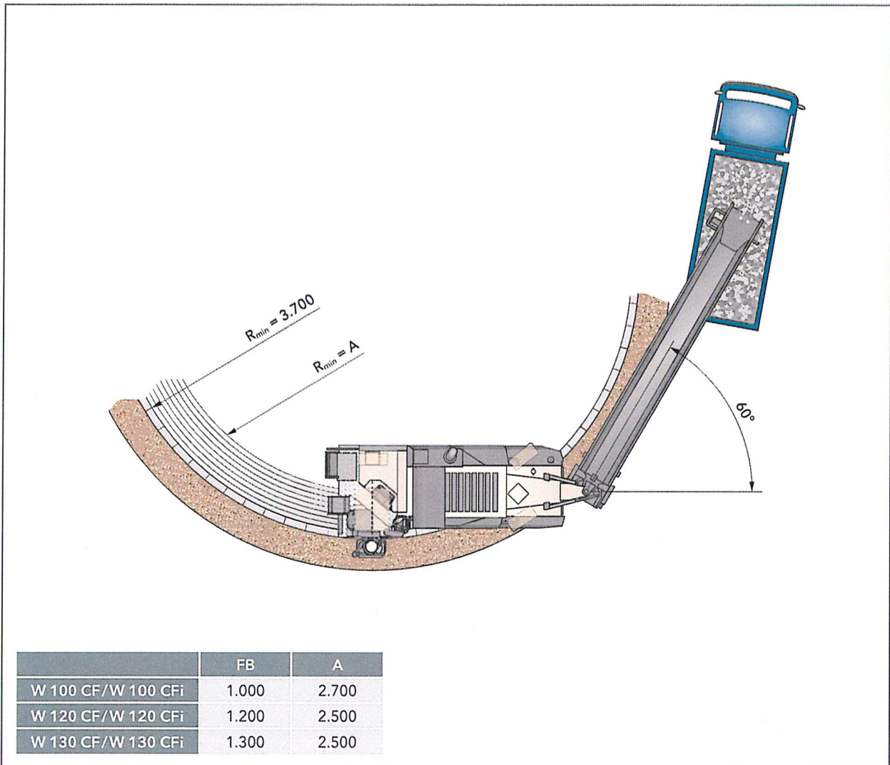
Fräskreis, Frästiefe 150 mm, Abmessungen in mm
